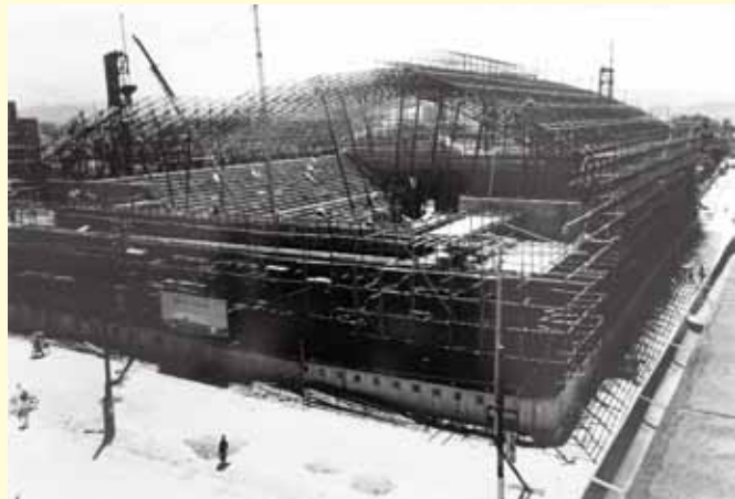
福岡スポーツセンター建設工事風景 屋根の輪郭が見えてきた建設工事をNHK福岡放送局階上より望む。 1955(昭和30)年9月頃 所蔵:西日本鉄道(株)
